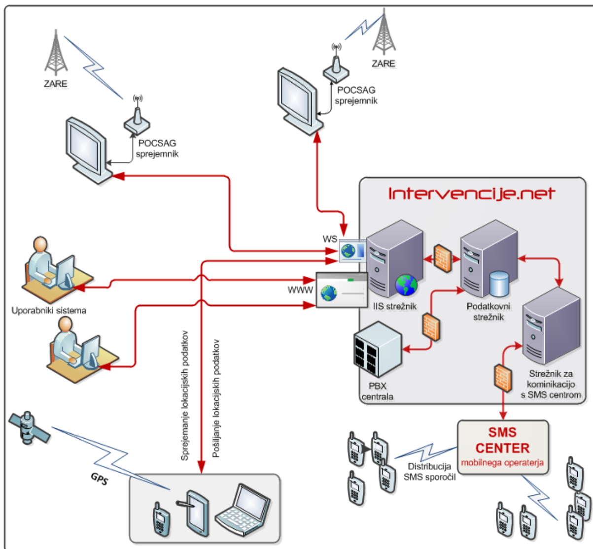
Slika 2 - Blok shema sistema Intervencije.net
